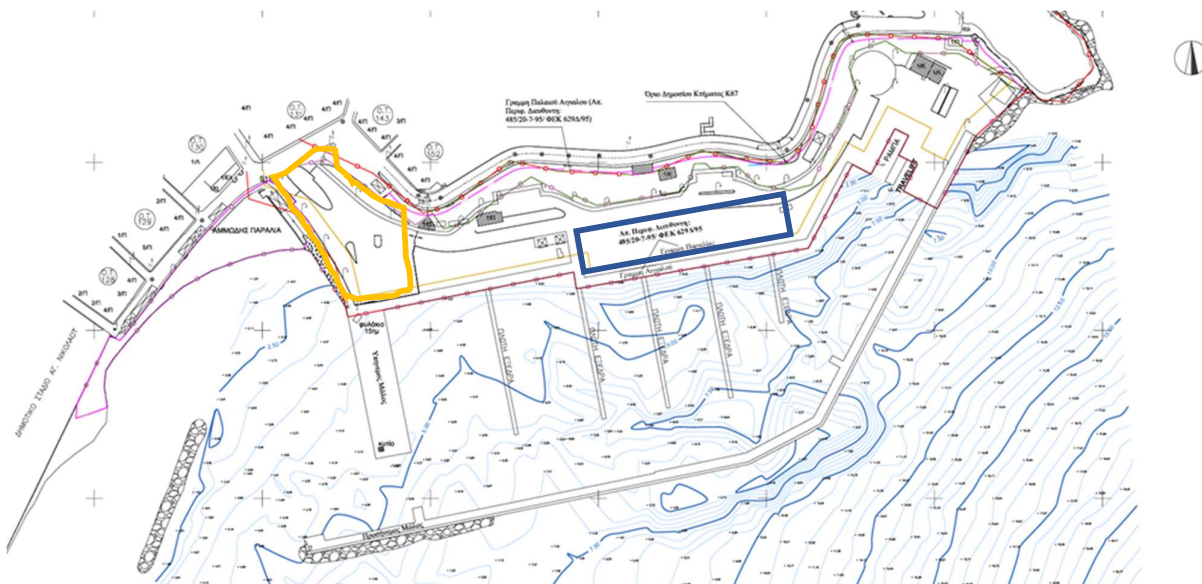
Σχ. 8 Χώρος διαχείμησης σκαφών (μπλε περιγραμμά)
