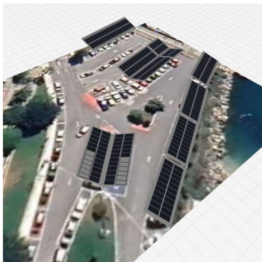
Εικόνα 5: Ενδεικτική χωροθέτηση φωτοβολταϊκού συστήματος με 250 ΦΒ πλαίσια συνολικής ισχύος 147,5 kWp.
